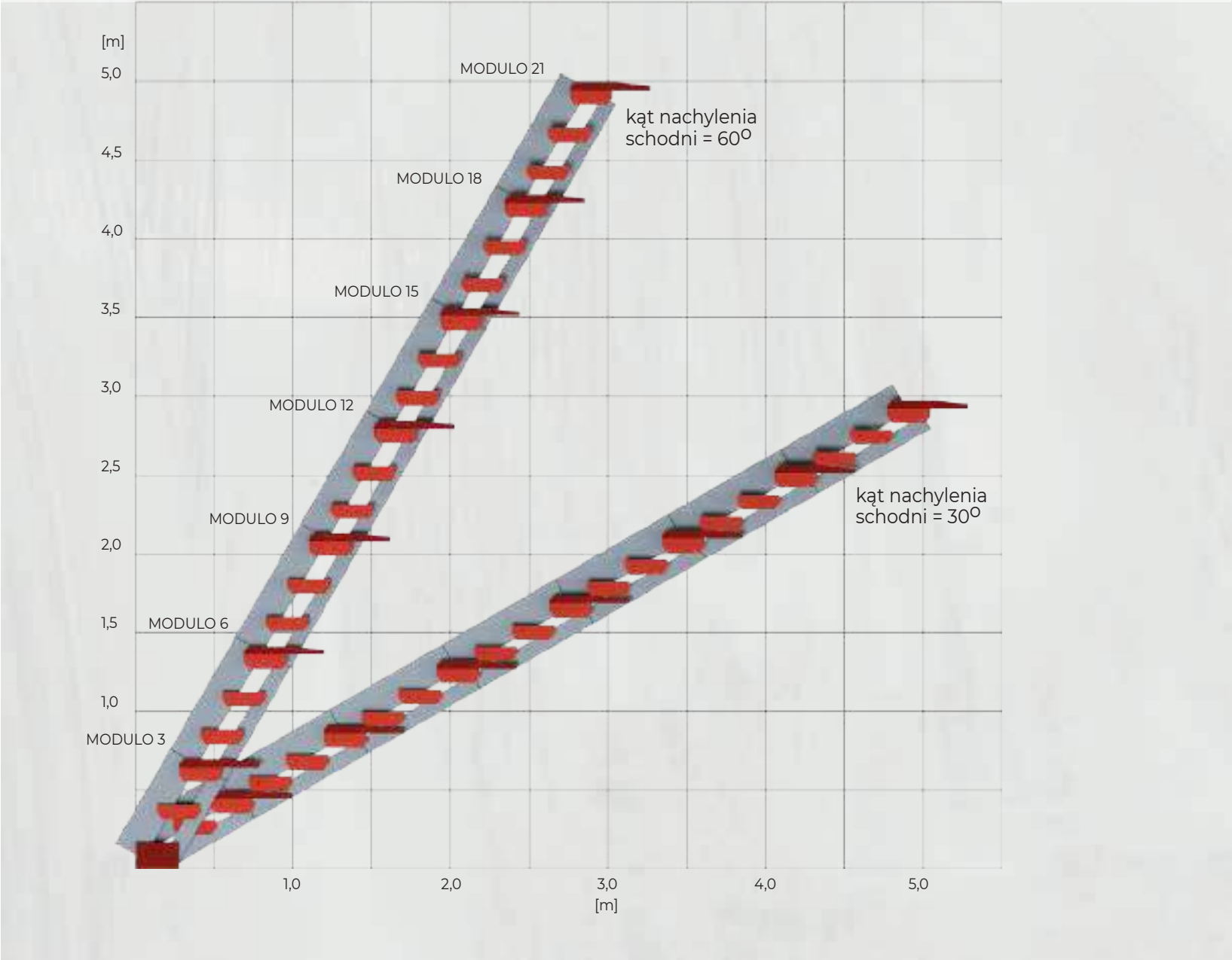
REGULACJA KĄTA NACHYLENIA SCHODNI
