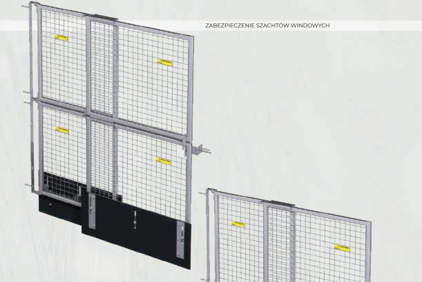
ZSW - SKRZYDŁO GÓRNE
