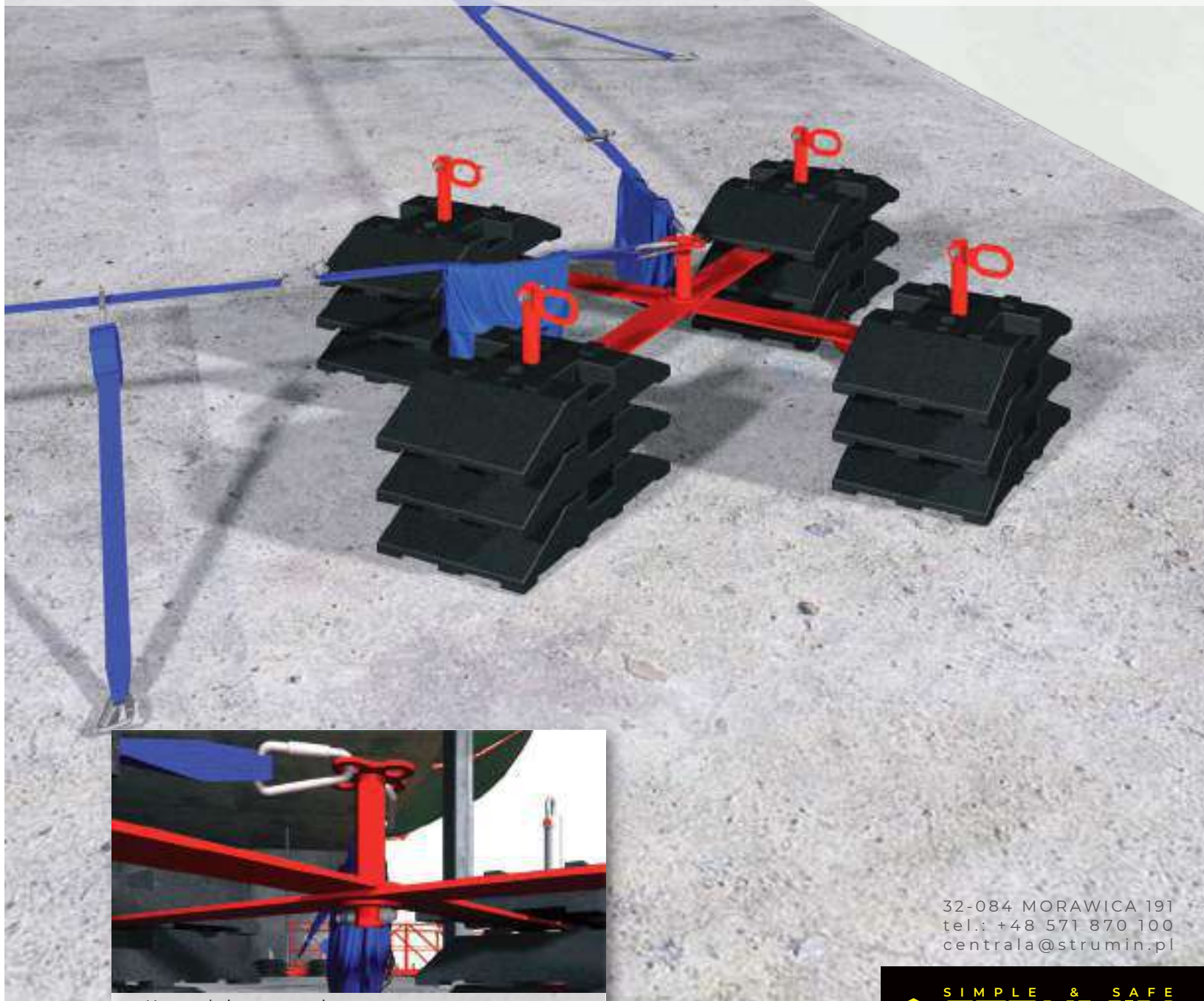
Konstrukcja amortyzująca.
